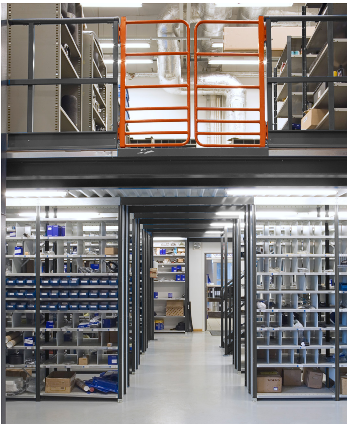
I ett plocklager kan entresolplanet byggas på EABs hyllställ. Här med en upplastningsplats med självstängande grind.
