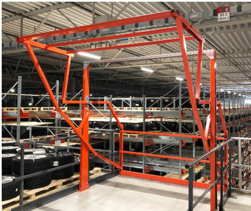
Upplastningsplats med vippgrind
